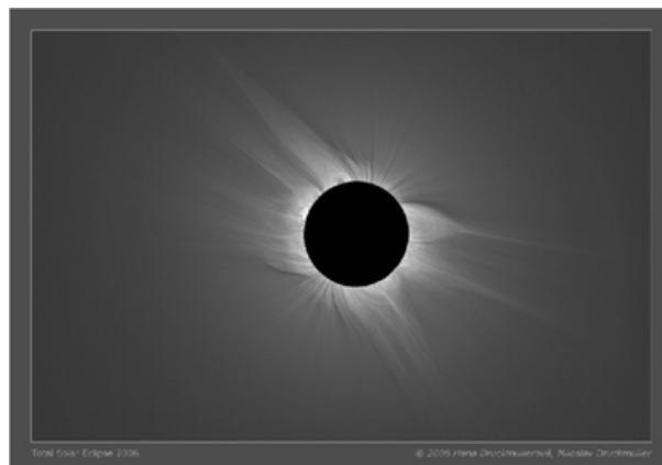
Obr. 10. Kompozice sluneční koróny pořízený ze snímků Hany Druckmüllerové z turecké Cappadocie
