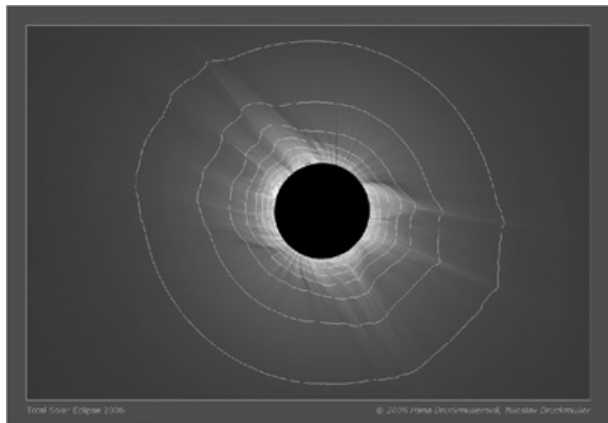
Obr. 13. Průběh izofot v koróně 29.3.2006
