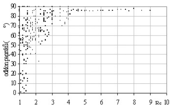
Obr. 14. Odklony koronálních struktur od radiálního směru
