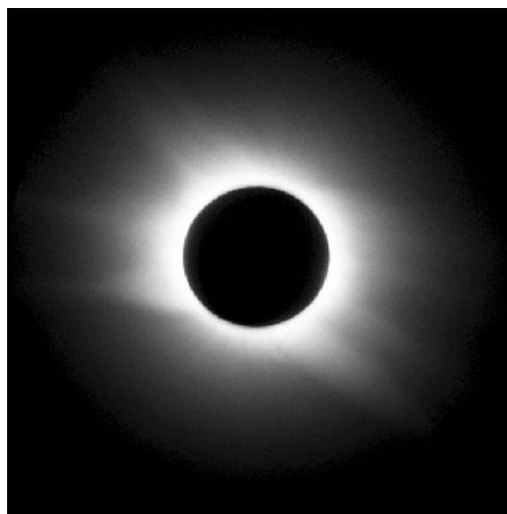
Obr. 7. Snímek pořízený objektivem MTO500 (1 s) v Egyptě
