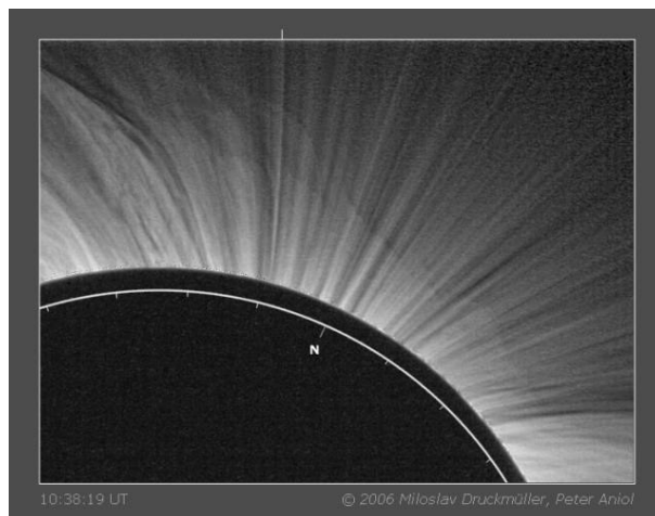
Obr. 13. Polární oblast s vyznačeným paprskem v P.A.350°
