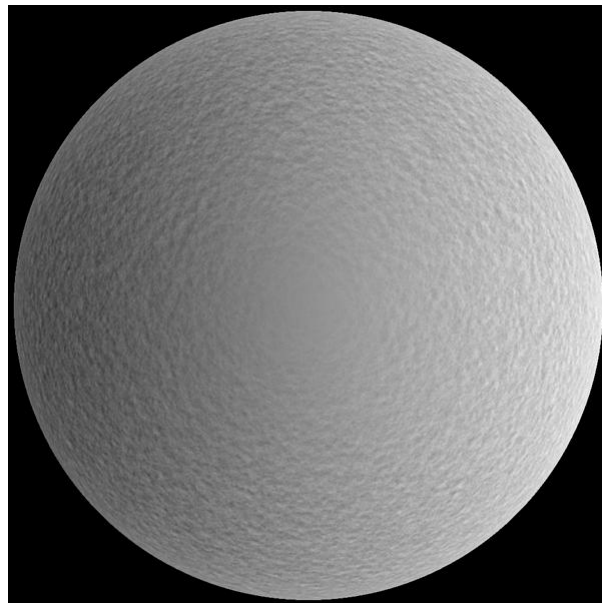
Obr. 1: Dopplerovské rychlostní pole slunečního disku včetně složky, vznikající rotací Slunce kolem své osy.
