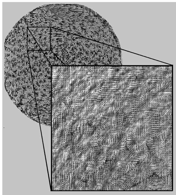
Obr. 3: Vektorové rychlostní pole pohybů hmoty v tenké vrstvě sluneční fotosféry. V popředí je zvětšený segment vektorového rychlostního pole, se superponovanou supergranulární sítí.
