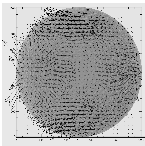
Obr.4: Velkostrukturální rychlostní pole pohybující se hmoty v tenké vrstvě sluneční fotosféry, získané prostorovou filtrací rychlostního pole celého slunečního disku na obr. 3. Vektory na okraji disku jsou zatíženy značnou chybou v důsledku průměrování i mimo disk.
