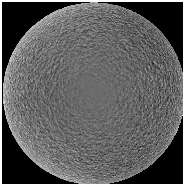
Obr. 2: Dopplerovská rychlostní pole na slunečním disku s odstraněnou složkou Carringtonovy rotace.
